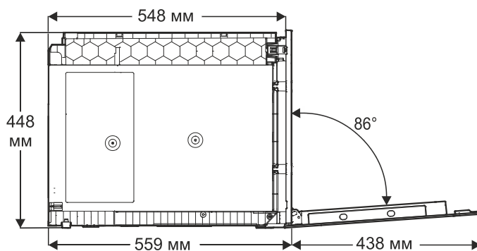
Вид сбоку
