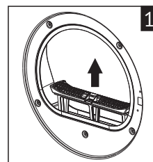
1. Entfernen Sie die Rückseite des Flusenfilters.
