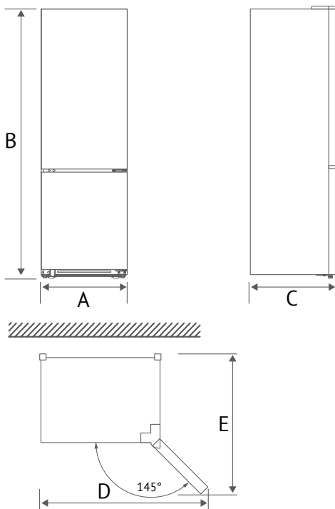
Схема требований минимального расстояния
