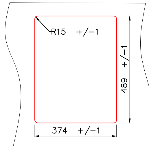
Врезной монтаж мойки (I)
