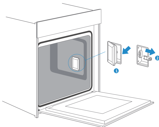
Боковая лампа
