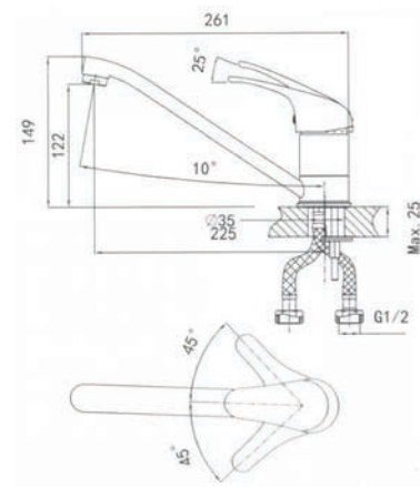
Размеры и установка
