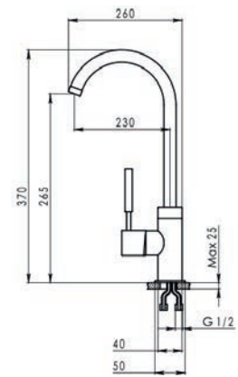
Размеры и установка
