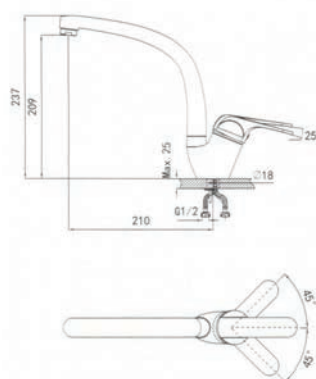
Размеры и установка
