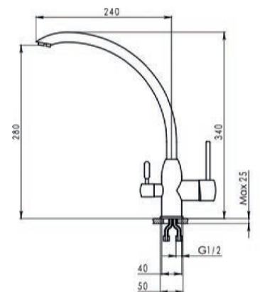
Размеры и установка
