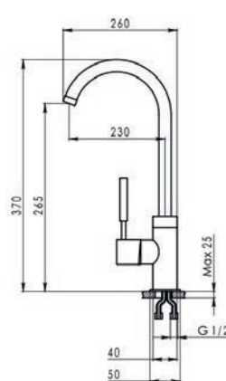
Размеры и установка
