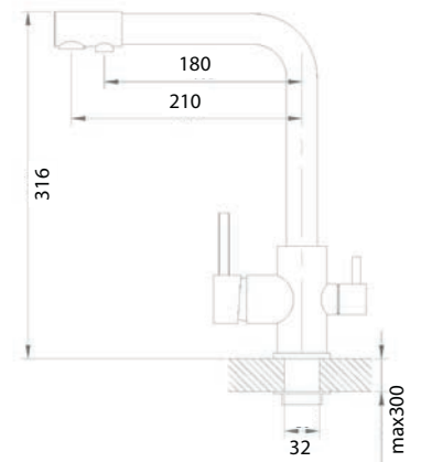
Размеры и установка
