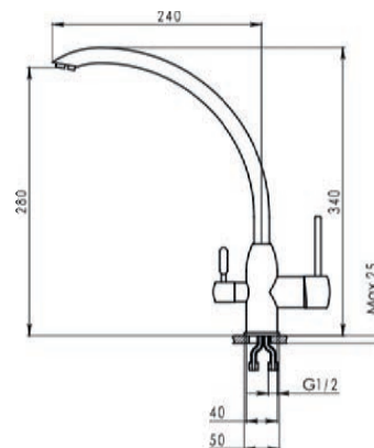
Размеры и установка
