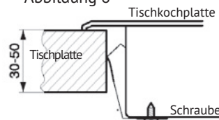
Befestigungsklammern
