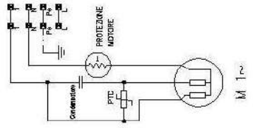
Schema funzionale COMPRESSORE
